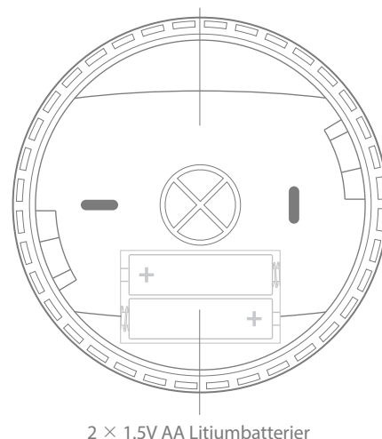
Monteringsplatta
